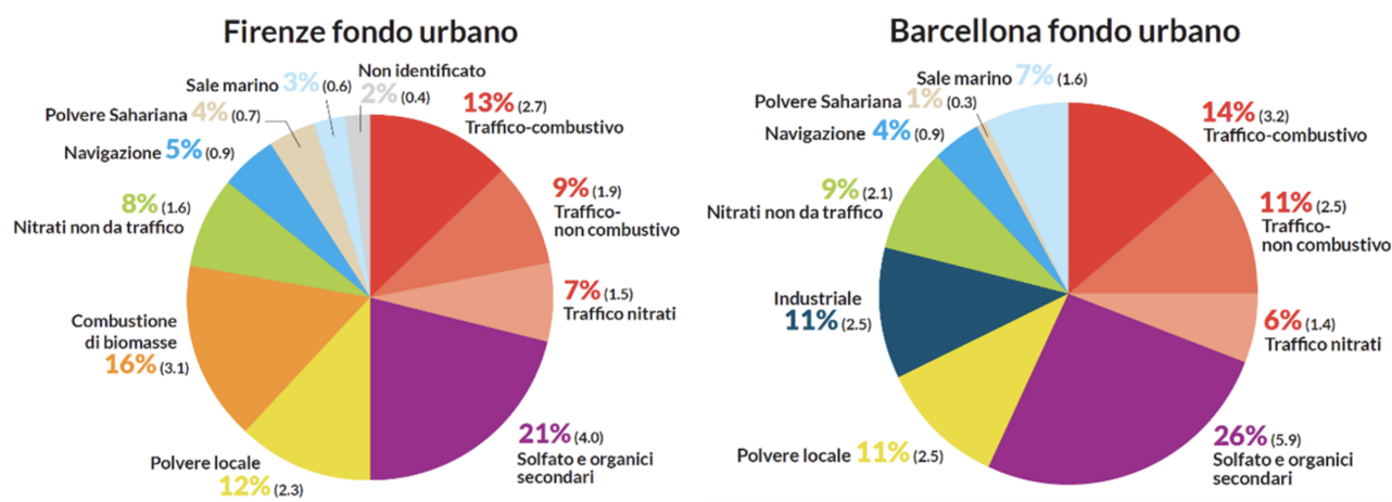
Figura 6: Contributo delle sorgenti al PM10, ottenuto tramite analisi PMF dei dati di composizione chimica del particolato a Firenze e Barcellona (media annua 2013-2014).
