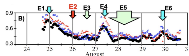
Figura 10: Andamento temporale del rapporto tra le concentrazioni orarie di Ca e Al nelle frazioni di particolato totale (senza taglio dimensionale), grossolana ( 2,5\text{--}10 \mu\text{m} ) e fine ( < 2,5 \mu\text{m} ) ottenuto all'Osservatorio di Izaña dal 23 al 30 agosto 17 [20]. Sono evidenziati i rapporti nel periodo in cui Izaña è stata interessata dal passaggio di aerosol proveniente dal Sahara.
