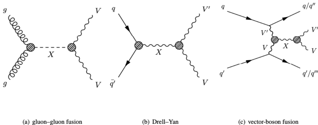
Figura 1: Diagrammi di Feynman che rappresentano la produzione di nuove particelle pesanti indicate con X con i loro decadimenti in una coppia di bosoni, indicati collettivamente come V : (a) fusione gluone-gluone, (b) Drell-Yan, (c) fusione vettore-bosone. I cerchi tratteggiati rappresentano gli accoppiamenti di X con le altre particelle, sia diretti che effettivi.
