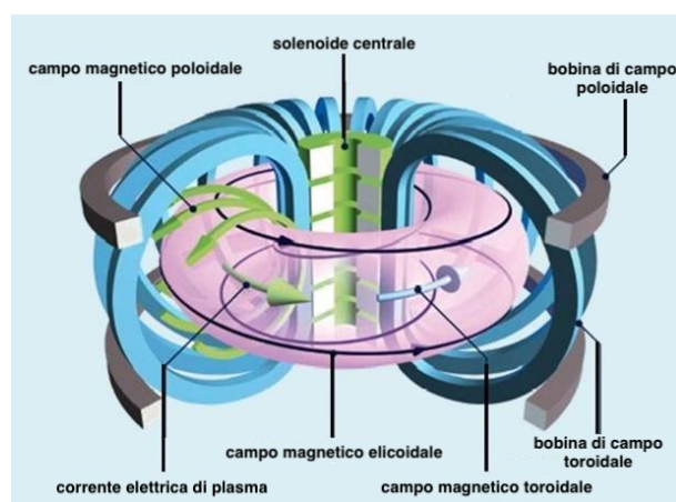
Figura 1: Illustrazione schematica del plasma confinato magneticamente in un tokamak (Immagine adattata dell'originale per cortesia di The Czech Academy of Sciences, Institute of Plasma Physics, con un ringraziamento speciale a UKAEA).
