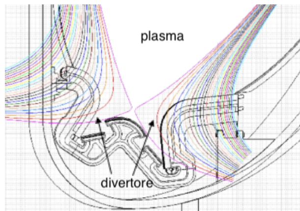
Figura 5: Illustrazione schematica del divertore nel Divertor Tokamak Test (DTT) [28, 29] (riproduzione da originale in Ref. [28]). Le superfici di flusso magnetico aperte sono rappresentate dalle linee colorate che confluiscono sulla struttura materiale del divertore. La regione di plasma è caratterizzata da superfici di flusso magnetico chiuse non indicate in figura.
