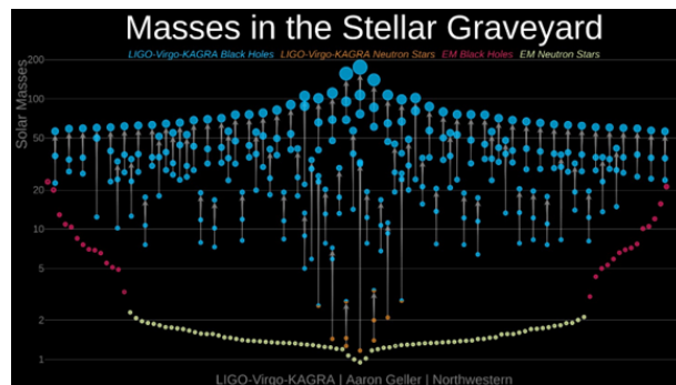
Figura 8: Stato della nostra conoscenza attuale di buchi neri di massa stellare e stelle di neutroni dopo i tre periodi di presa dati dei rivelatori di onde gravitazionali dal 2015 al 2020. Ogni insieme blu contiene tre punti: le masse (in unità di masse solari, scala in ordinata) dei buchi neri prima della fusione, e la massa del buco nero dopo la fusione. Le masse dei buchi neri conosciute prima dell'avvento degli interferometri per onde gravitazionali sono in rosso (a sinistra e destra). L'esistenza di buchi neri di massa > 20 masse solari era inaspettata prima dell'avvento di questi strumenti. I pochi punti in arancio in basso sono invece le coalescenze di stelle di neutroni, e i punti in giallo in basso sono le stelle di neutroni la cui massa era stimata tramite l'osservazione delle onde elettromagnetiche. Crediti: LIGO-Virgo / Aaron Geller / Northwestern University.
