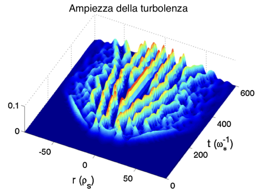
Figura 2: Andamento spazio-temporale dell'ampiezza della turbolenza di deriva. La scostamento nella coordinata radiale r rispetto alla posizione iniziale del pacchetto d'onda è espresso in unità del raggio di Larmor ionico calcolato alla temperatura degli elettroni, \rho_s . Il tempo è espresso in unità dell'inverso della frequenza diamagnetica, \omega_*^{-1} . (Immagine adattata dall'originale di Ref. [14]).
