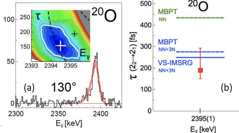
Figura 5: Pannello a sinistra: Spettro per la transizione \gamma a 2396 keV dallo stato a lunga vita lungo ( \tau = 3.5 \text{ ps} ) nel nucleo ^{20}\text{O} misurato con lo spettrometro AGATA (con precisione < 4 \text{ mm} ) a 130^\circ . Lo spettro simulato sovrapposto ai dati corrisponde al minimo valore della differenza tra lo spettro misurato e quelli simulati in corrispondenza a diversi valori del tempo di vita dello stato e dell'energia della transizione gamma. Pannello a destra: Valore della vita media misurata confrontato con diverse previsioni teoriche. Quelle che includono l'interazione a tre corpi riproducono meglio il valore sperimentale. Figura tratta da referenza [2].
