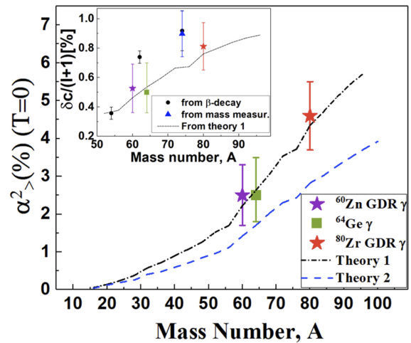
Figura 9: Miscelazione isospin \alpha^2 e correzione miscelazione isospin \delta_c in funzione del numero di massa calcolati utilizzando teorie basate sui funzionali densità energia (DFT). Stelle e quadrati sono valori sperimentali ottenuti utilizzando transizioni di tipo E1 che sono proibite nel caso non ci sia la rottura della simmetria di isospin. Figura tratta da referenza [2].
