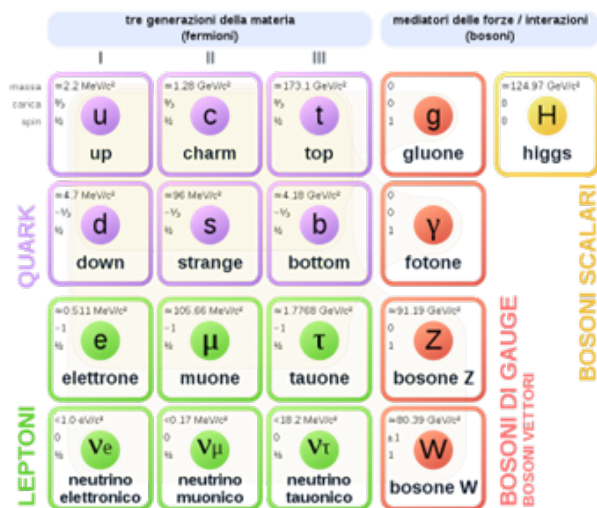
Figura 1: Tabella riassuntiva del modello standard delle particelle elementari, con i costituenti ultimi della materia, in base alle nostre conoscenze. Per ogni particella è riportata massa, carica e spin. A sinistra, le tre generazioni della materia (o famiglie di particelle) che sentono le interazioni. La prima famiglia (I) contiene l'elettrone e il suo neutrino e i quark u e d di cui sono costituiti protone e neutrone. Le tre famiglie di particelle hanno in corrispondenza tre famiglie di antiparticelle. A destra, le particelle che scambiano le interazioni. Per queste, non sussiste distinzione tra particella e antiparticella.
