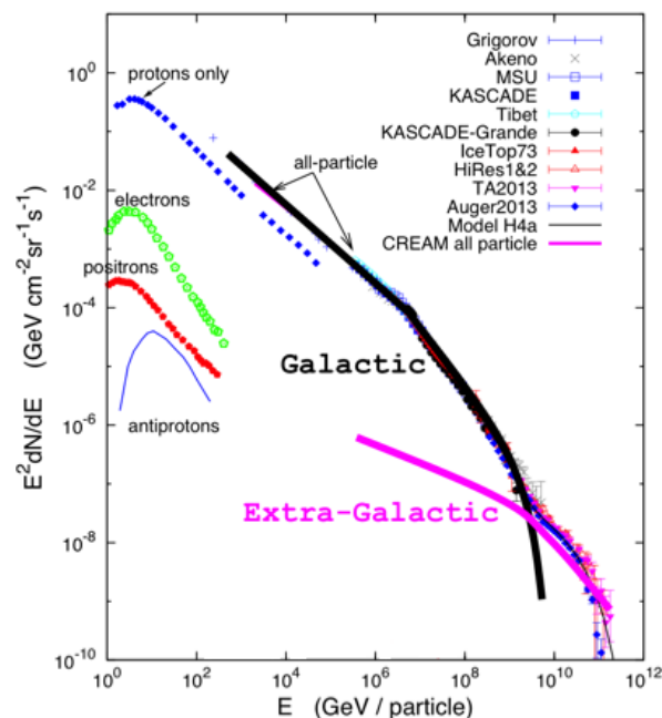
Figura 3: Flusso di raggi cosmici (RC) in arrivo sulla Terra in funzione dell'energia. I RC sono particelle stabili, in prevalenza protoni e nuclei, accelerati da sorgenti galattiche ed extragalattiche. Le due curve (nera e viola) rappresentano i contributi relativi di queste due componenti. La frazione di elettroni nei RC (punti verdi) è minoritaria. Gli elettroni non riescono a sfuggire dalle regioni di accelerazione a causa dei meccanismi di perdita di energia. Nei RC sono presenti anche antiparticelle: positroni (ossia, anti-elettroni punti rossi) e antiprotoni (linea blu). Queste anti-particelle sono prevalentemente prodotte dall'interazione dei RC con il mezzo interstellare. La figura è presa da una compilazione didattica della Collaborazione IceCube utile da consultare [4].
