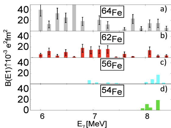
Figura 7: Intensità delle transizioni di tipo dipolare misurata con il rivelatore AGATA per i nuclei ^{62,64}\text{Fe} e con fasci radioattivi. Figura tratta da referenza [2].
