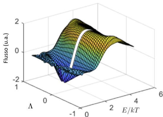
Figura 4: Flusso di particelle (in unità arbitrarie) nello spazio delle fasi ridotto utilizzato per descrivere le strutture zonali nello spazio delle fasi. Le coordinate rappresentano due degli integrali primi che caratterizzano il moto di singola particella nell'equilibrio magnetico. Figura riprodotta con permesso da Ref. [30].
