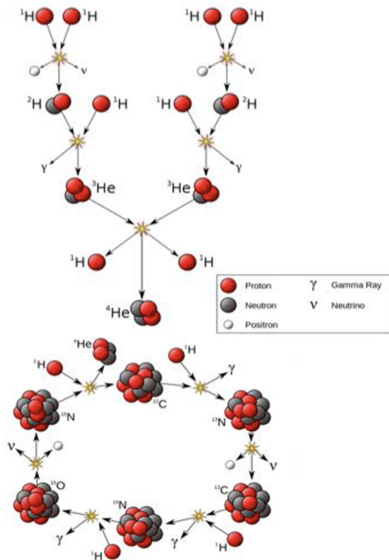
Figura 2: Illustrazione schematica del ciclo dell'idrogeno, parte superiore, e del CNO (Carbonio, Azoto, Ossigeno) nella parte inferiore.
