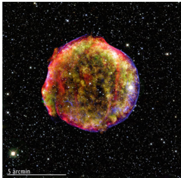
Figura 2: Questa immagine mostra la regione dove avvenne l'esplosione di una stella brillante testimoniata da Tycho Brahe e altri astronomi di quell'epoca (1574). L'immagine combina osservazioni a raggi X e infrarossi ottenute rispettivamente con l'Osservatorio a raggi X Chandra della NASA e il telescopio spaziale Spitzer, e all'Osservatorio di Calar Alto, in Spagna. Tutta l'emissione è dovuta al moto di elettroni nella regione in cui sono presenti intensi campi magnetici. Crediti: Raggi X: NASA/CXC/SAO, Infrarossi: NASA/JPL-Caltech; Ottico: MPIA, Calar Alto. [3]
