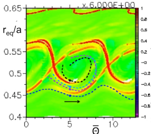
Figura 3: Interazione risonante onda-particella descritta attraverso il codice girocinetico HM-GC. Sono rappresentate diverse traiettorie di particelle nello spazio delle fasi individuato dalla coordinata radiale (normalizzata al raggio del plasma a ) e dalla fase onda-particella \bar{\theta} . Le traiettorie sono sovrapposte alla struttura risonante prodotta dalle fluttuazioni elettromagnetiche mostrata come curve di livello dei "Finite time Lyapunov exponents" del sistema. Figura riprodotta con permesso da Ref. [24].
