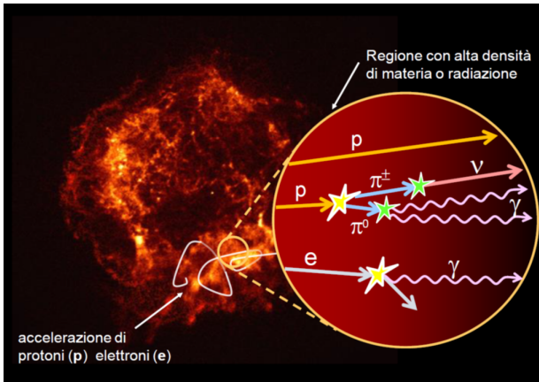
Figura 4: Interconnessione tra raggi cosmici (RC), raggi gamma ( \gamma ) e neutrini ( \nu ). Sorgenti astrofisiche possono accelerare RC (protoni, elettroni e nuclei) a enormi energie. Gli elettroni dissipano gran parte della loro energia localmente. Una frazione dei protoni e nuclei diffonde all'esterno della regione di accelerazione, si propaga nello spazio galattico (o intergalattico, se la sorgente è esterna alla Galassia) e può giungere sulla Terra. I RC carichi non viaggiano in linea retta a causa delle deflessioni dovute a campi magnetici. La misura della direzione di arrivo dei RC non permette quindi di determinare la posizione della sorgente. Una frazione di protoni (o nuclei) accelerati può invece interagire con la materia o coi campi elettromagnetici che circondano la sorgente. In questo caso, il decadimento di particelle secondarie neutre (principalmente \pi^0 ) produce una coppia di raggi- \gamma , mentre il decadimento di particelle cariche (principalmente \pi^+ oppure \pi^- ) produce neutrini. L'interazione di elettroni con la materia o radiazione produce solo raggi- \gamma . Quindi, la rivelazione di neutrini dalla direzione di una sorgente è un modo univoco per scoprire quali sono le sorgenti acceleratrici di protoni e nuclei.
