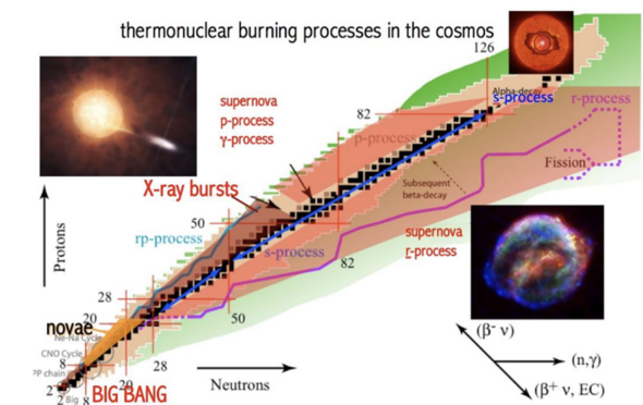
Figura 1: Illustrazione schematica della carta dei nuclidi con indicazione dei diversi processi di nucleosintesi.
