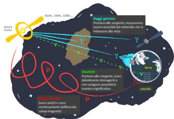
Figura 5: Schema di propagazione dalle possibili sorgenti (nella galassia o extragalattiche) alla Terra di raggi cosmici carichi (principalmente, protoni), raggi gamma e neutrini. Raggi gamma e neutrini sono particelle neutre e si propagano in linea retta, ma hanno caratteristiche di propagazione differenti. Immagine: Juan Antonio Aguilar and Jamie Yang. IceCube/WIPAC (adattata in italiano).
