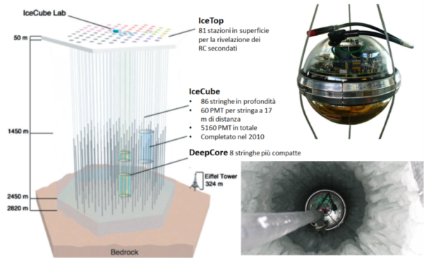
Figura 6: Schema del rivelatore IceCube al Polo Sud. Oltre ad una matrice di rivelatori posti a grande profondità sotto il ghiaccio, sono visibili anche dei rivelatori posti sopra la superficie. Nella foto a destra: in alto uno dei moduli ottici inseriti nel ghiaccio, con un PMT e l'elettronica necessaria per il funzionamento. In basso, uno dei buchi perforati nel ghiaccio con l'inserimento di una delle stringhe. Cortesia della collaborazione IceCube.
