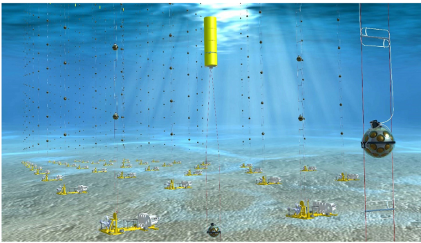
Figura 7: Vista sottomarina di un blocco del telescopio KM3NeT. Un blocco è composto da 115 stringhe. Ciascuna stringa consiste di 18 moduli ottici (la sfera che si vede in primo piano a destra). Ciascuna sfera contiene 31 PMT, i piccoli occhi elettronici che captano la luce. La distanza verticale tra i moduli ottici è di circa 36 m, la distanza orizzontale tra le stringhe di circa 90 m. Appoggiato al fondo marino alla profondità di 3500 m vi è un'ancora per ciascuna stringa. Ogni stringa (700 m di altezza) viene tenuta in tensione da una boa gialla, una delle quali è ben visibile nella parte centrale. (Disegno di Edward Berbee/ Nikhef). Si ricordi che a 3500 m di profondità l'assorbimento della luce solare è praticamente totale. Un telescopio analogo, ma con stringhe e sfere più ravvicinate è in costruzione al largo delle coste di Tolone (Francia) con l'obiettivo di studiare le proprietà fisiche del neutrino. Cortesia della collaborazione KM3NeT.
