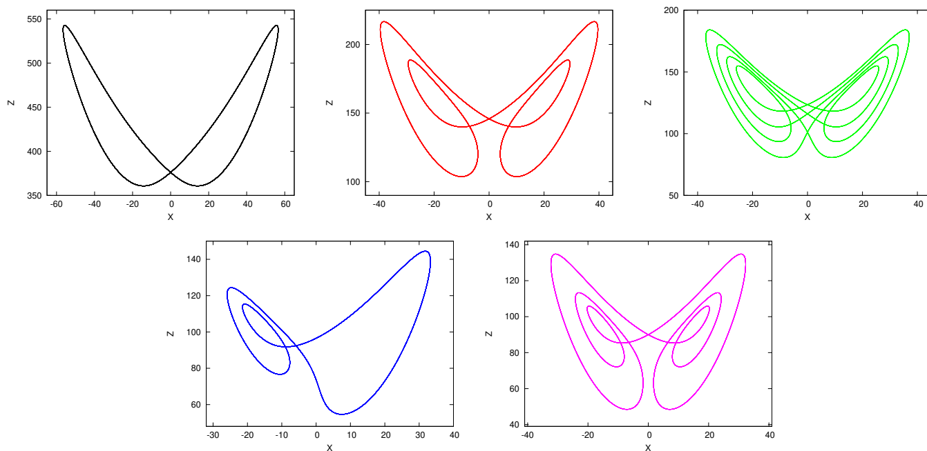
Figura 15: Proiezione dell'orbita sul piano (x, z) per \epsilon = 0.015 (prima finestra periodica, colore marrone); \epsilon = 0.025 (seconda finestra periodica, colore rosso); \epsilon = 0.02745 (terza finestra periodica, colore verde); \epsilon = 0.03152 (quarta finestra periodica, colore blu); \epsilon = 0.0328 (quinta finestra periodica, colore viola). Le coordinate x e z sono quelle del SdL nella forma originaria.
