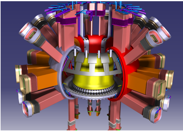
Figura 12: Immagine del divertore di DTT
